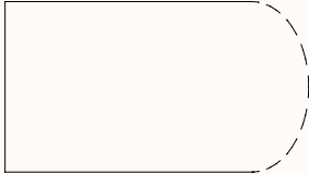
D-end Top OW 1200-2400mm OD 900-1200
